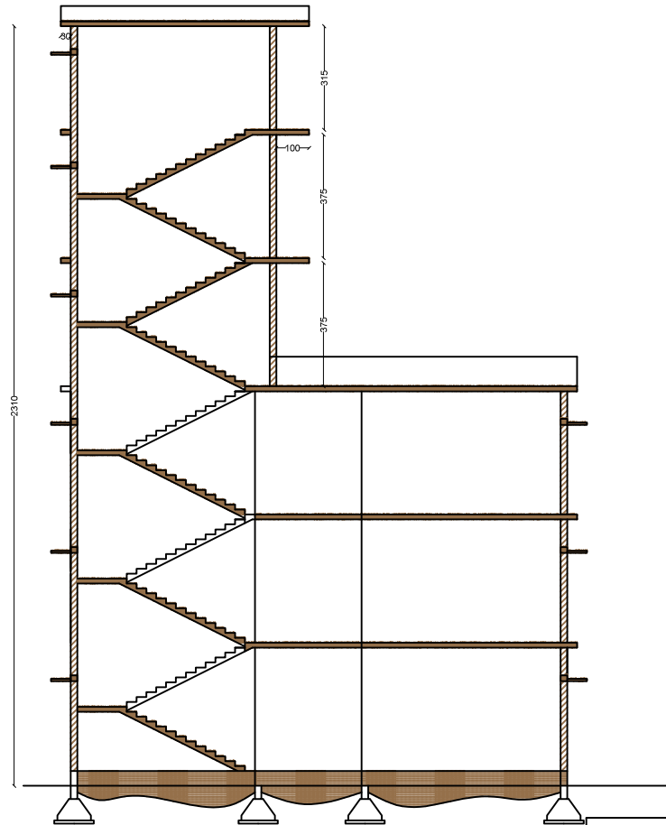
SECTION A-A
