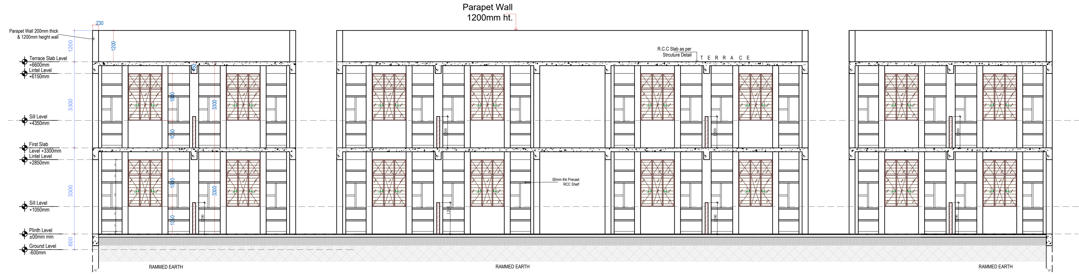
SECTION A-A
