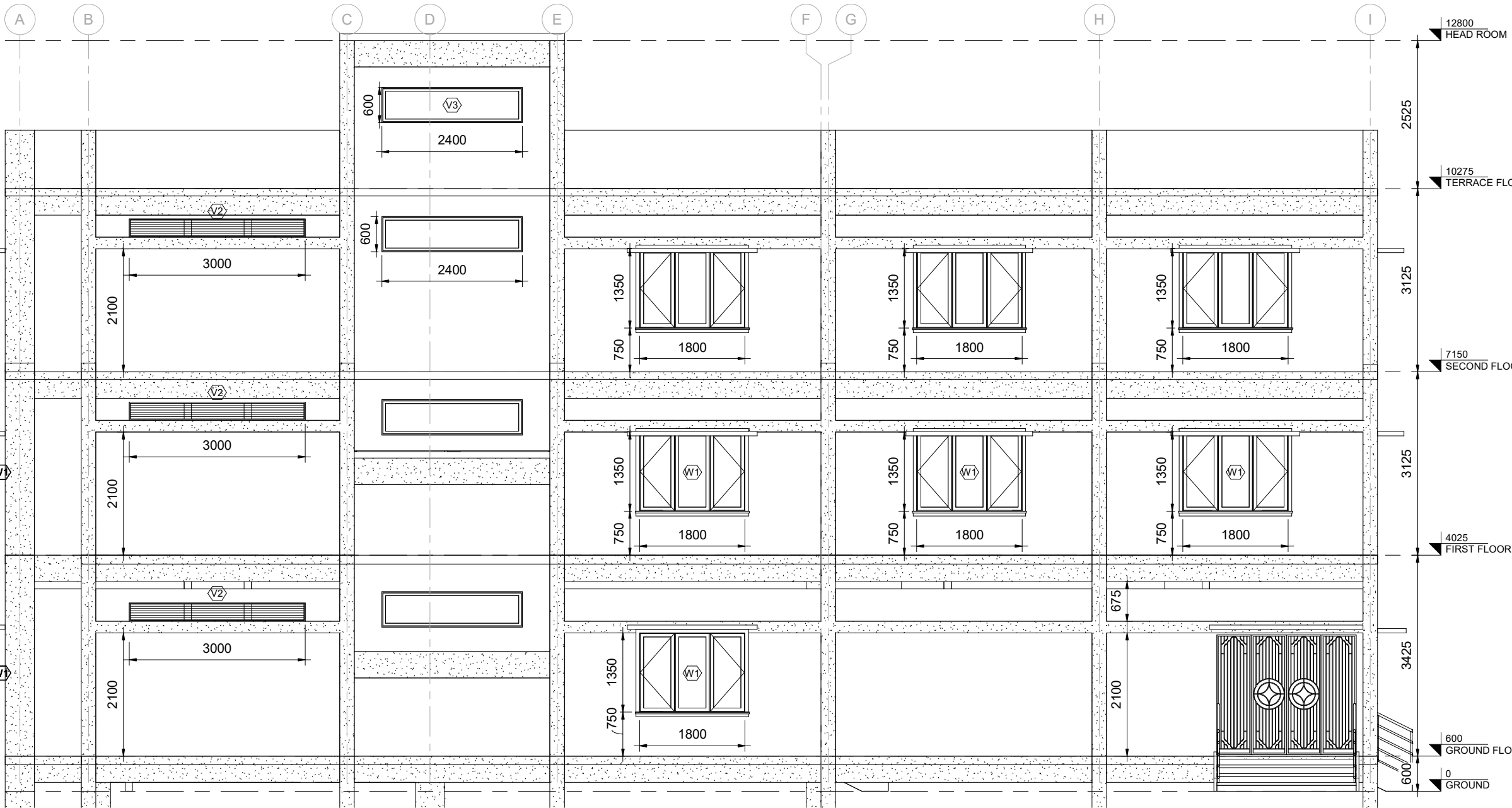
1 RIGHT ELEVATION 1 : 40
