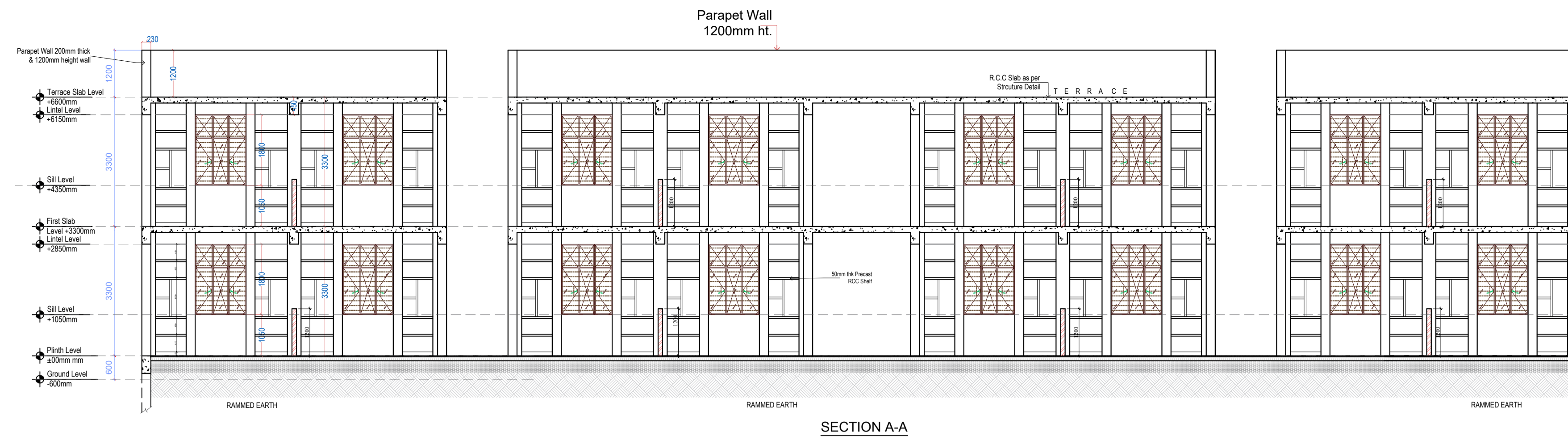
SECTION A-A
