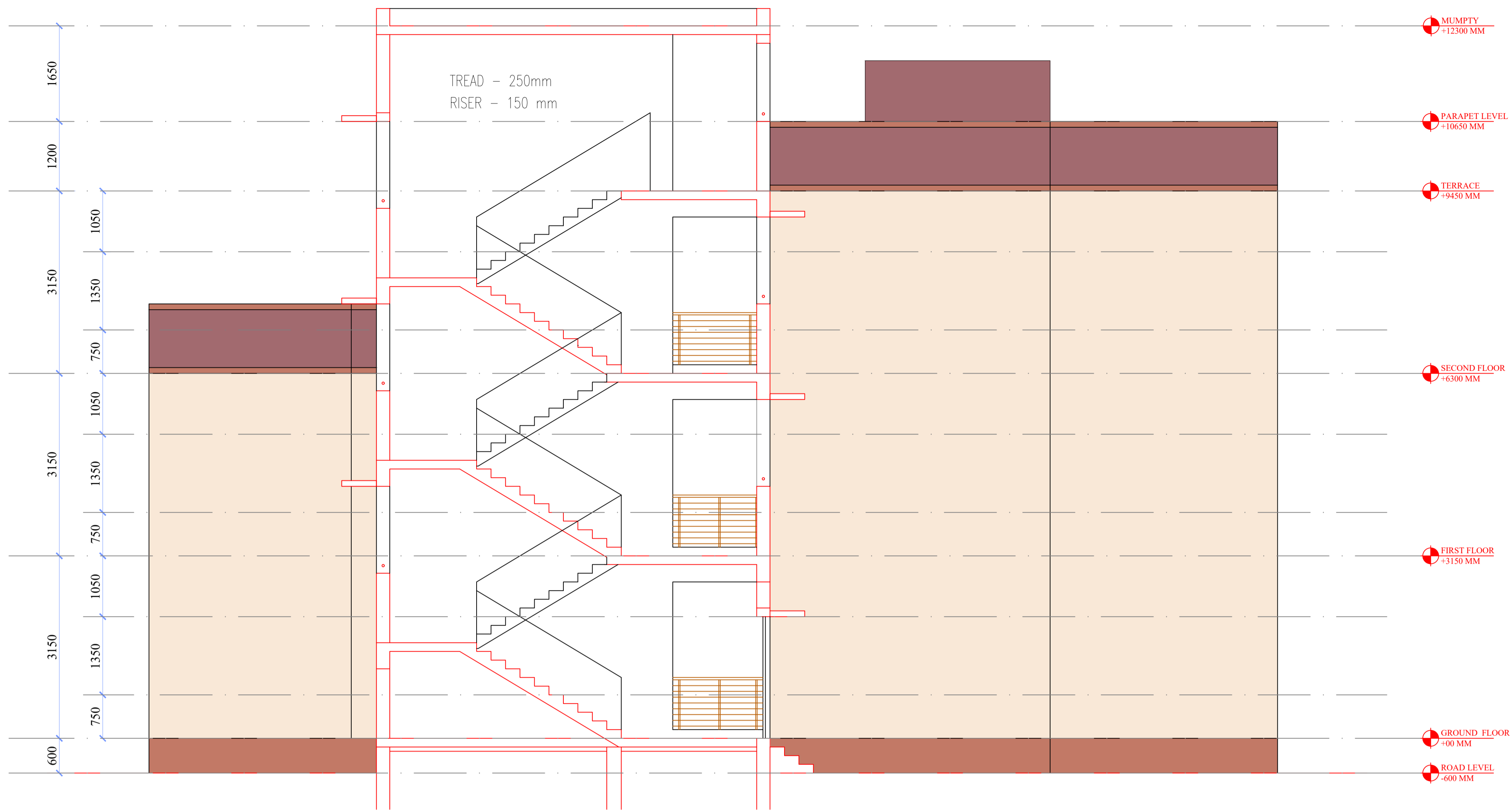
SECTION : S1
